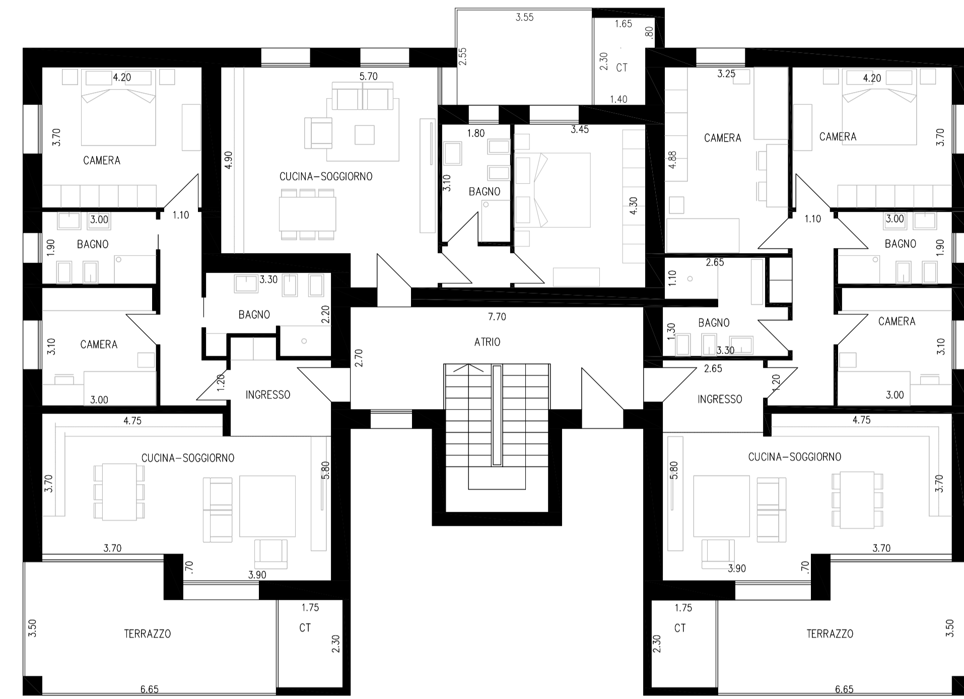
PIANO PRIMO
